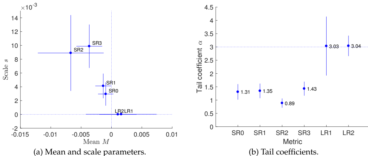
Figure 5: Parameter estimates
